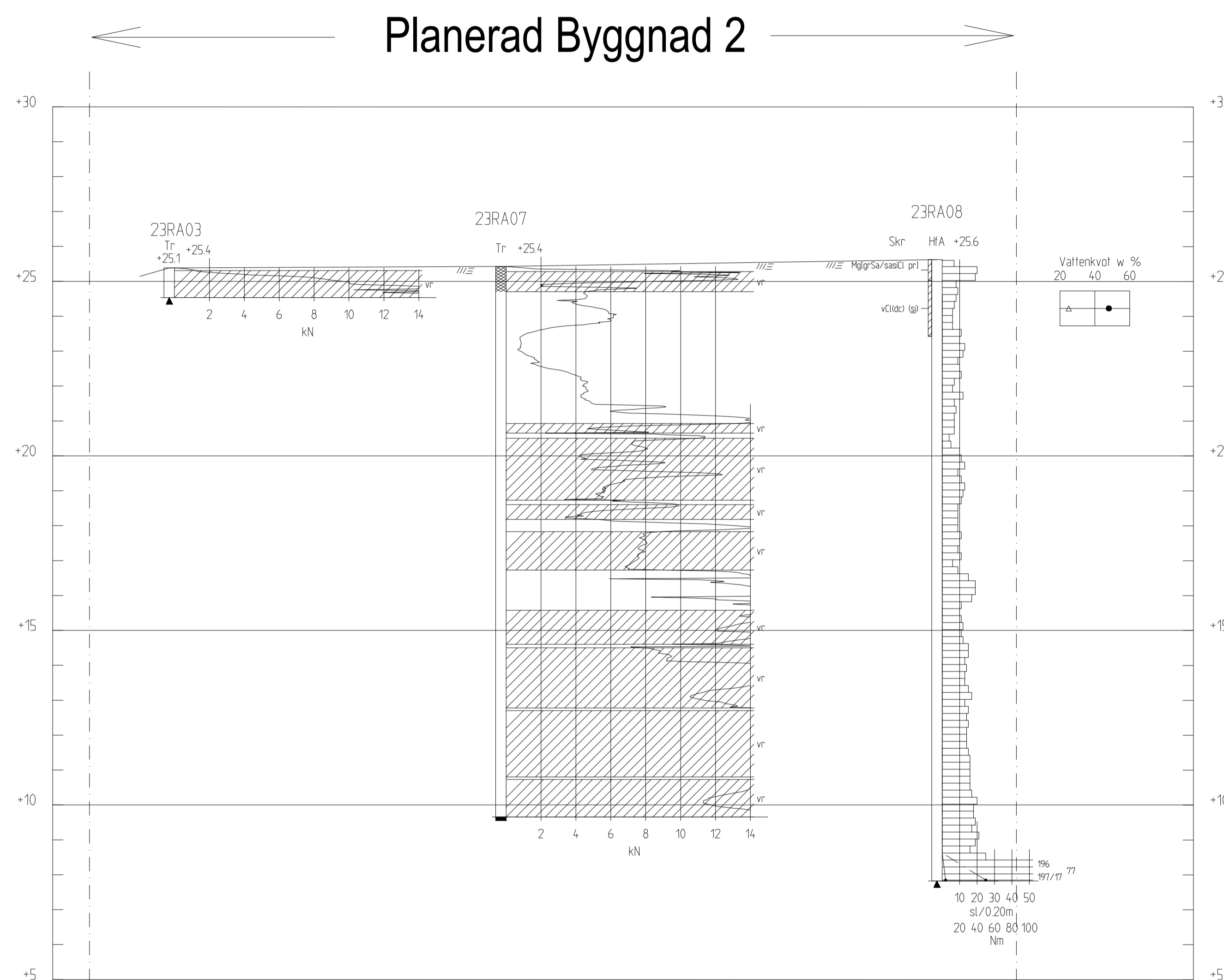
SEKTION G-G H 1: 100 L 1: 200
