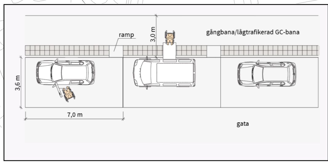
Illustration för långgående parkeringsplats för rörelsehindrade (kantstenspärning) från Uppsala kommun teknisk handbok.
