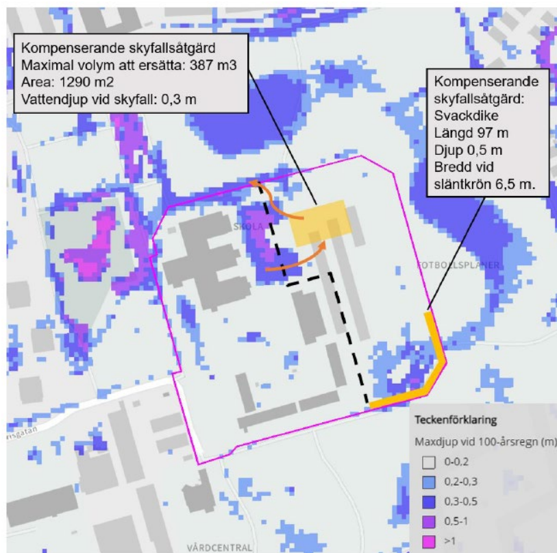
Figur 33 Befintliga lågpunkter inom planområdet enligt Uppsala vattens skyfallskartering tillsammans med planerade byggrätt (svart streckad linje). Gula områden markerar kompenserande åtgärder för skyfall. Observera att utbredning av åtgärderna motsvarar ett värsta scenario, d.v.s att lågpunkterna helt fylls igen. Exakt placering och utformning av skyfallsåtgärderna behöver utredas i kommande projektering då byggplanerna inom planområdet kommit längre.
