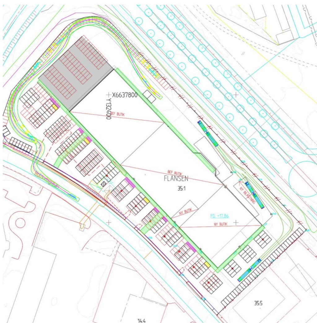
Figur 9 Situationsplan med föreslagen parkeringslösning för blandad handel. Föreslagen tillbyggnad redovisas i grått. Totalt 228 parkeringsplatser ryms inom fastigheten. Cykelparkering redovisas som rosa ytor.
