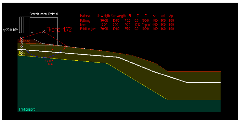
Figur 5. Stabilitetsberäkning.
