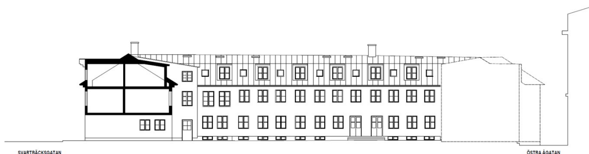
Fasaden på hus B mot gården (ritning: AQ 3 arkitektur).
