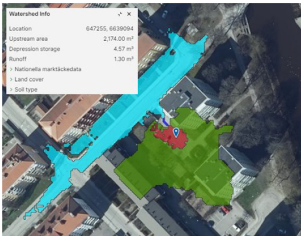
Bild 19. Flygfoto visar stående vatten inom fastigheten vid ett skyfall, beräknat för ett 100-årsregn. Illustration: PE Teknik & Arkitektur
