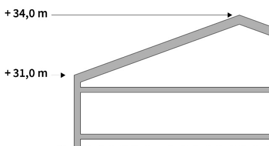
Bild 23. Sektion som illustrerar maximala höjder för nockhöjd respektive takfotshöjd.
