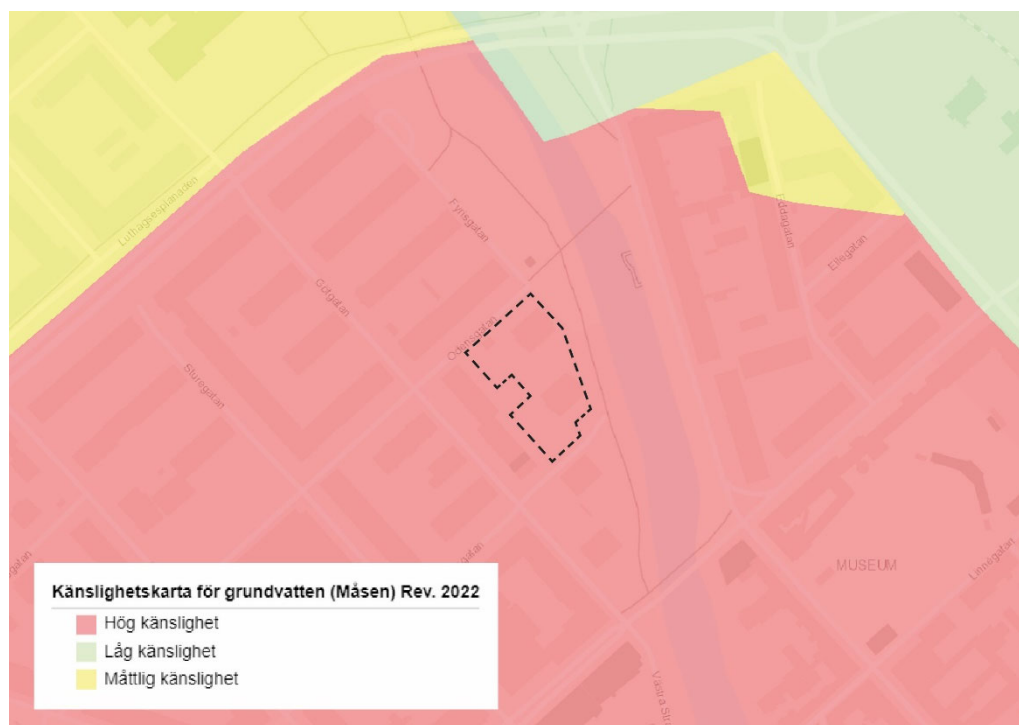
Bild 15. Utdrag från karta som visar grundvattnets känslighet (revidering 2022) som visar att planområdet ligger inom hög känslighet för påverkan på grundvattnet. Planområdet är markerat med en streckad linje.
