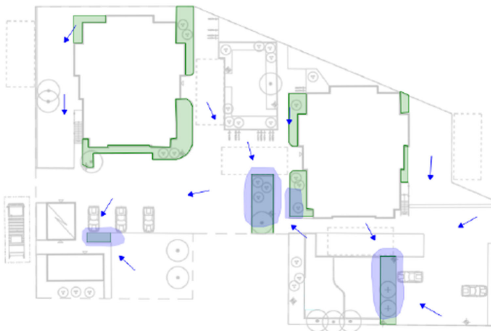
Bild 13. Illustrationsplan som visar föreslagen dagvattenhantering. Förslag på yttlig dagvattenavrinning visas med blå pilar och placering av växtbäddar är markerade i mörkgrönt. Förslag på områden där det vid skyfall skulle kunna bli stående vatten på ytan visas i mörkblå. Illustration: PE Teknik & Arkitektur
