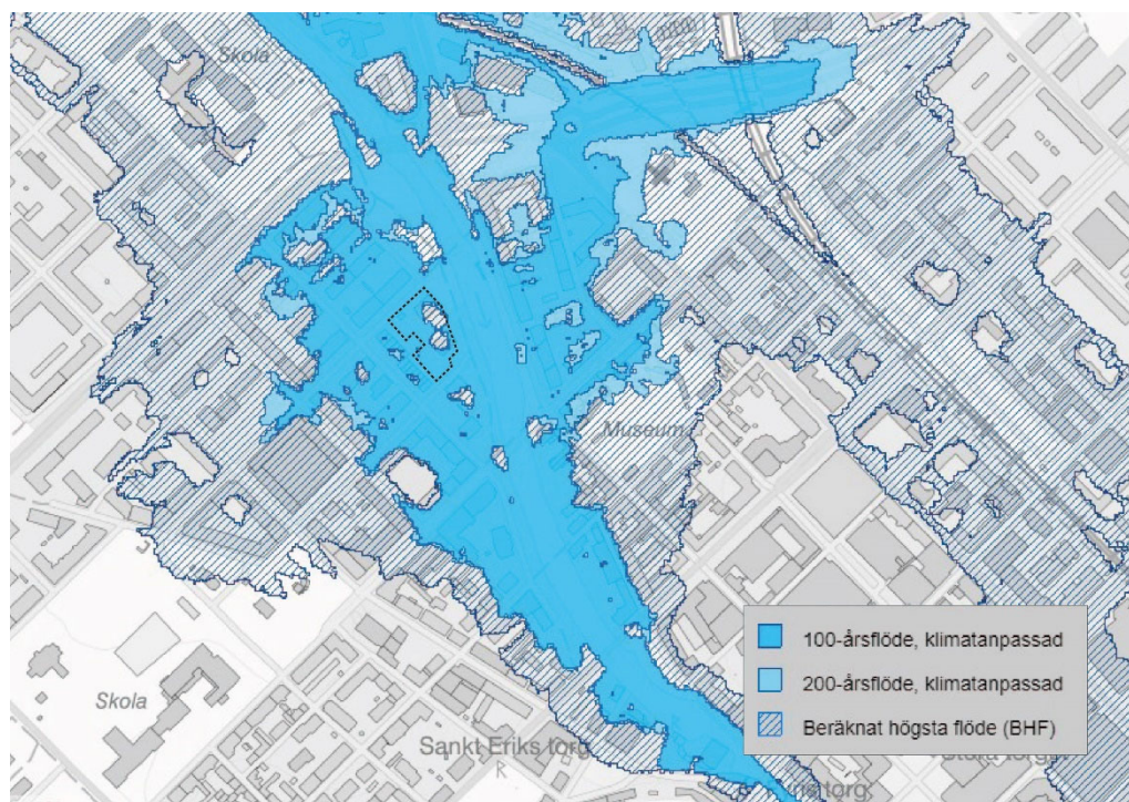
Bild 16. Karta från översvämningsportalen som visar hur planområdet kan komma att översvämmas av Fyrisåns 100- och 200-årsflöde, samt vid beräknat högsta flöde. Planområdet är markerat med en streckad linje.
