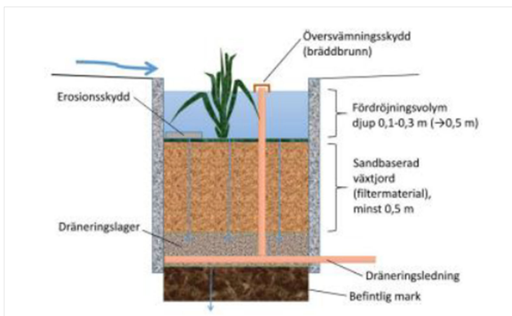
Bild 14. Sektion som visar utformningen av de växtbäddar som dagvattenutredningen föreslår ska anläggas för rening och fördröjning av dagvatten. Illustration: PE Teknik & Arkitektur
