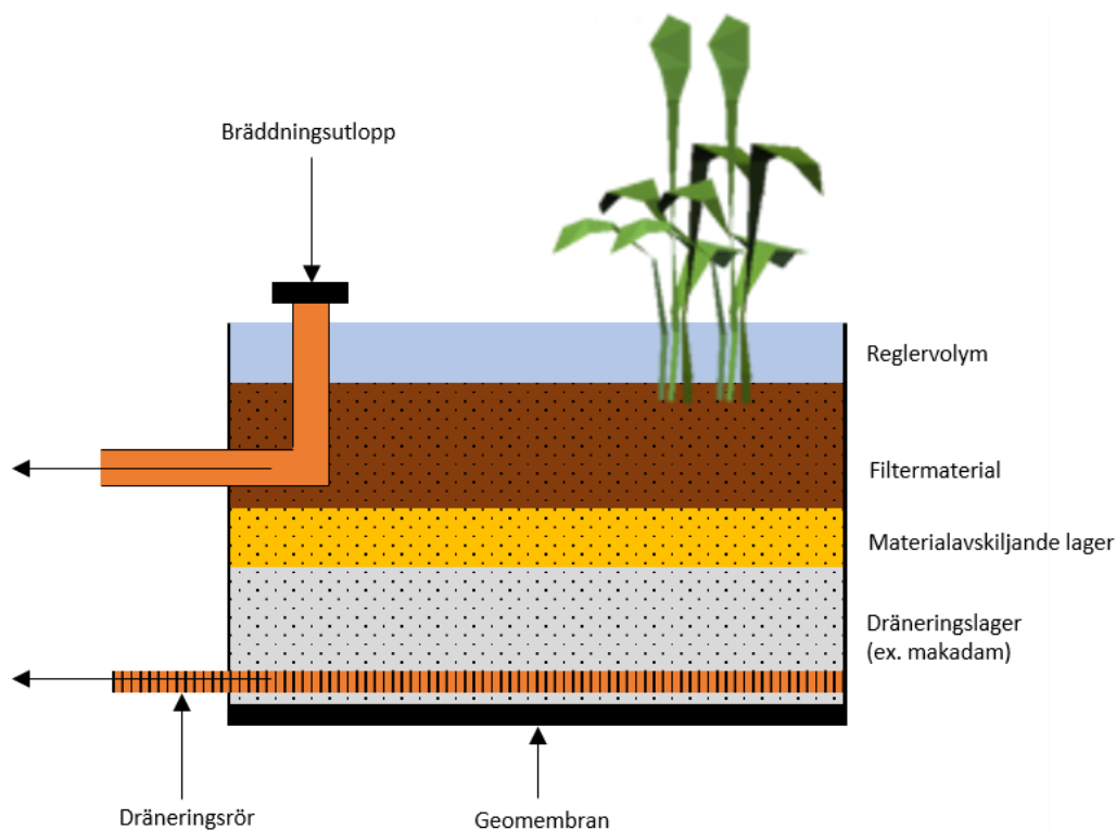
Figur 6-3. Principskiss över uppbyggnad av en regnbädd efter Payne m.fl. (2015). I exemplet tillåts inte dagvatten infiltrera i underliggande mark utan leds till befintligt dräneringssystem.
