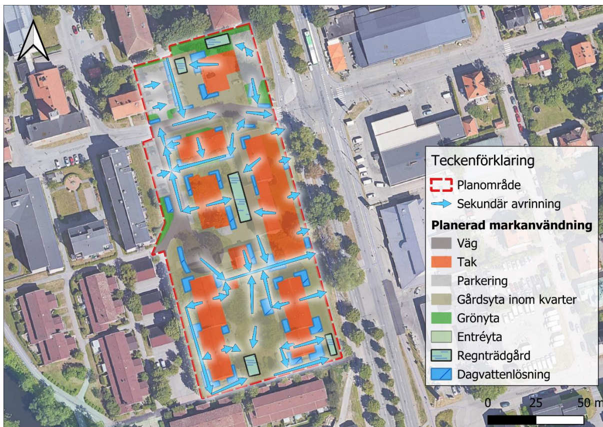
Figur 7-2. Planområdets höjdsättning ska medföra att dagvattnet rinner bort från byggnadernas fasader och ut från innergården i händelse av skyfall. Dessa avrinningsvägar kallas sekundära avrinningsvägarna och de blå pilarna anger rekommenderad flödesriktning.
