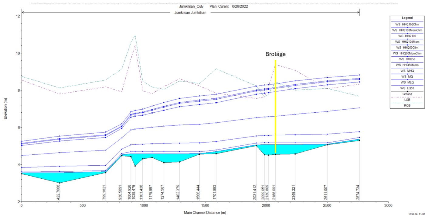
Figur 4: Beräknade vattennivåprofiler (blå linjer) för olika flöden (nedifrån räknat LLQ, MLQ, MQ, MHQ, HQ50 och HQ100) vid bro läget. Svart linje visar bottennivåer i vattendraget och gul linje ungefärligt bro läge.
