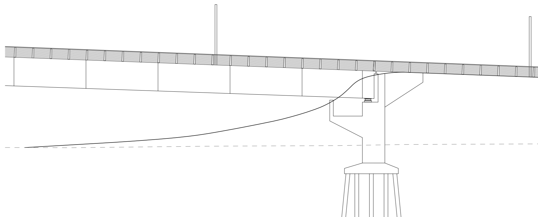
Längdsektion landfäste
