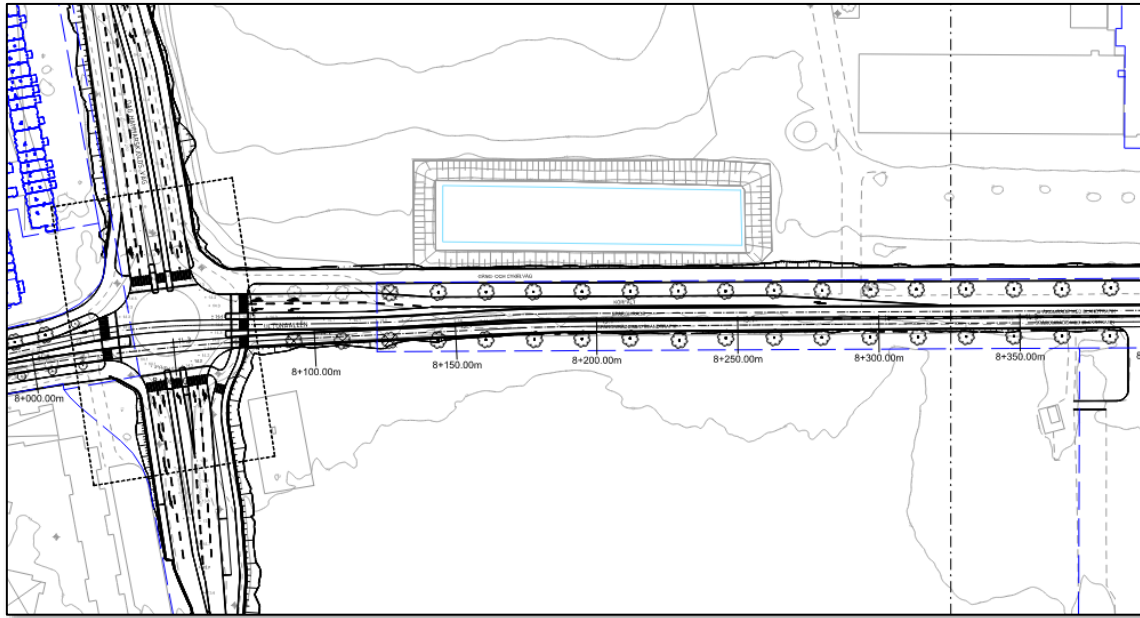
Figur 15. Föreslagen spårdragning med blandtrafik längs Ulltunaallén, öster om Dag Hammarskjölds väg, med befintlig bebyggelse i grundkarta.
