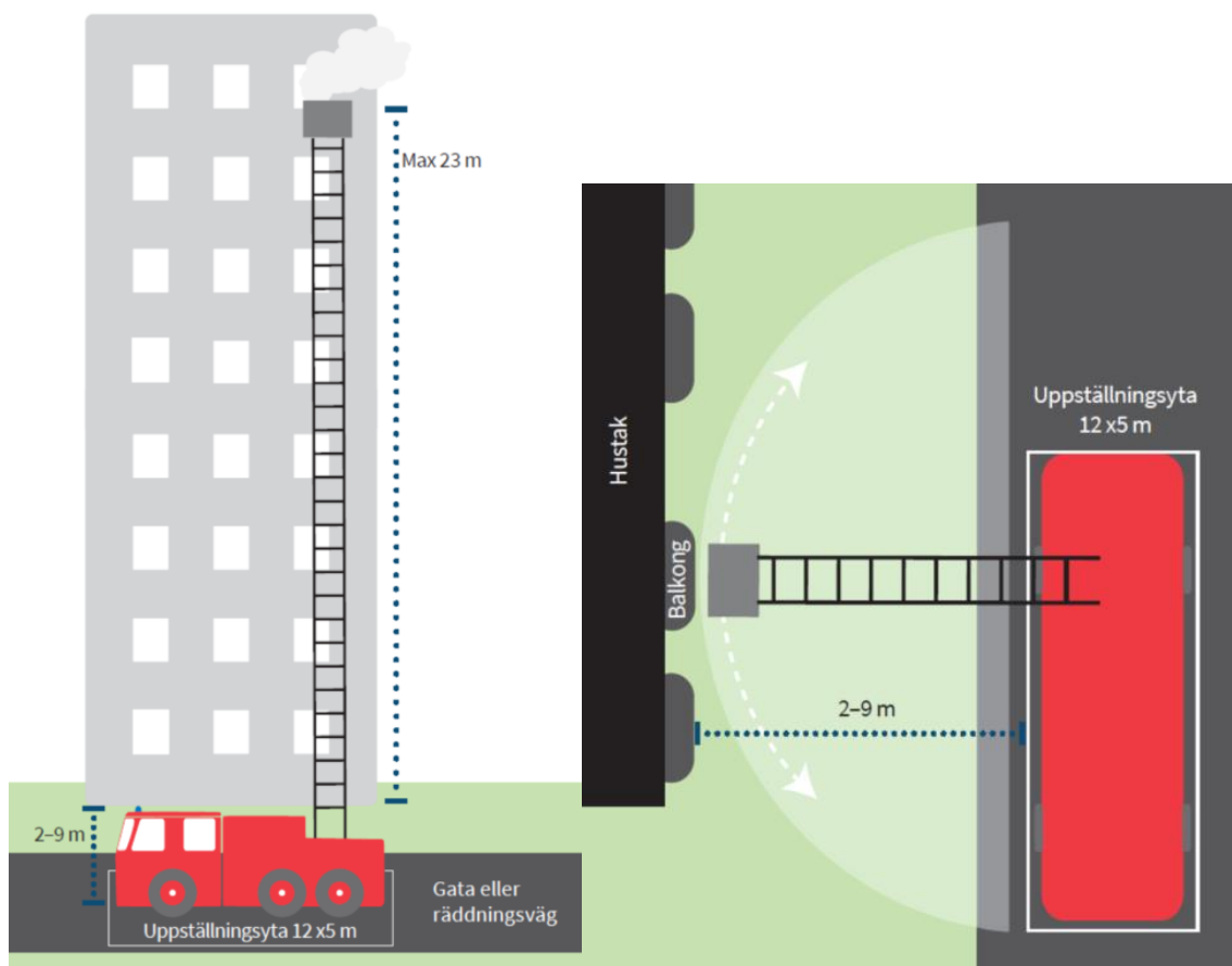
Figur 10. Förutsättningar för utrymning med höjdfordon. Fritt avstånd från fasad till höjdfordonet om 2–9 meter medför ett behov om fri uppställningsplats om 7-14 meter från fasad (inräknat fordonets bredd om 5 meter). Uppsala Brandförsvaret rekommenderar att avståndet bör vara minst 11 meter fritt avstånd från fasad (6 meter plus fordonets bredd) för att ge goda förutsättningar vid manövrering av höjdfordonets korg.
