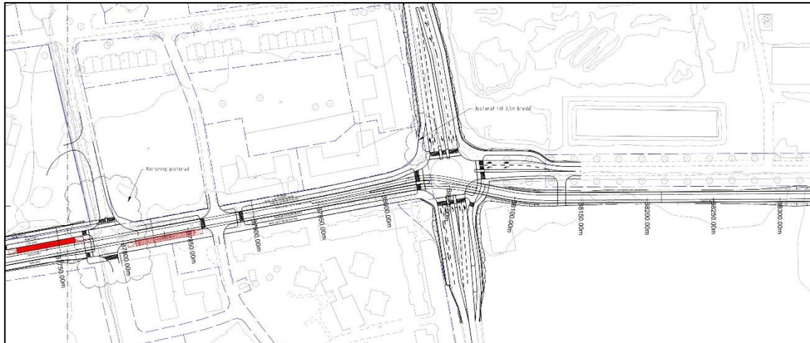
Figur 13. Föreslagen spårdragning med befintlig bebyggelse i grundkarta.
