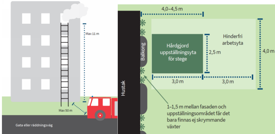
Figur 11. Förutsättningar för utrymning med bärbar stegutrustning.
