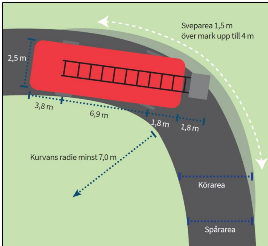
Figur 21. Dimensionering av kurvor för ett typfordon.
