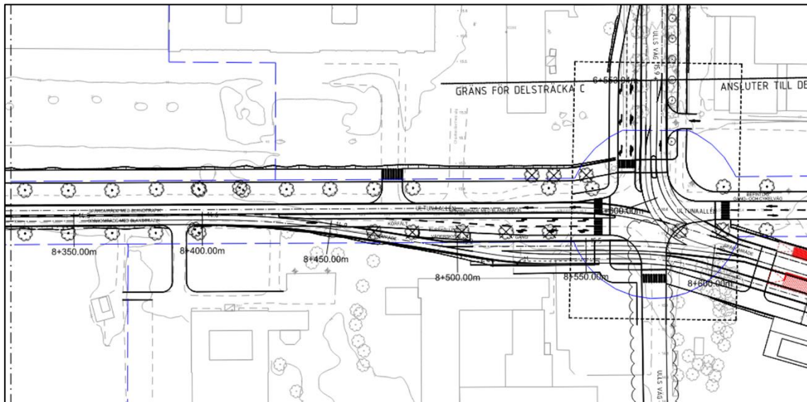
Figur 16. Föreslagen spårdragning med blandtrafik längs Ulltunaallén, väster om Ulls väg, med befintlig bebyggelse i grundkarta.
