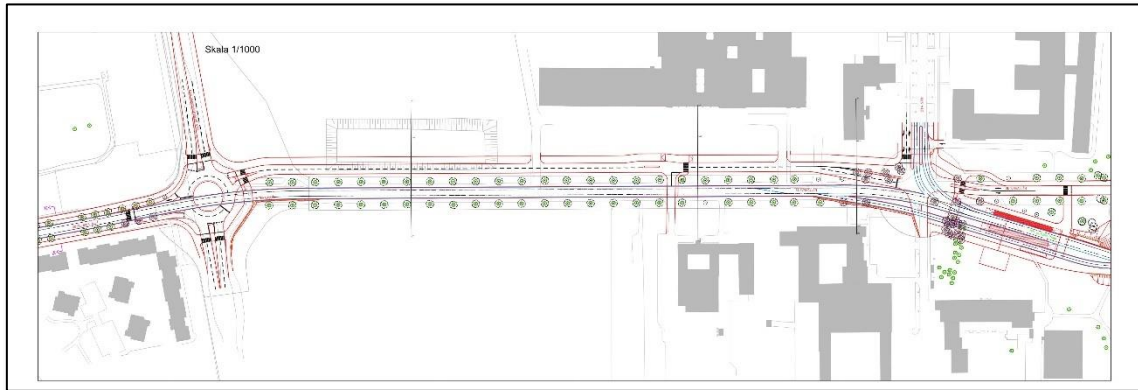
Figur 17. Utrett alternativ med Ulltunaallén i ett nytt nordligt läge. Alternativet innebär en cirkulationsplats i korsningen Ulltunaallén/Dag Hammarskjölds väg.
